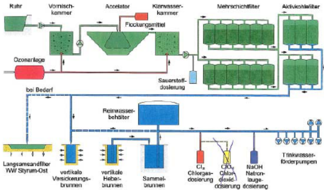
Fließschema der Wasseraufbereitung WW Styrum-West
