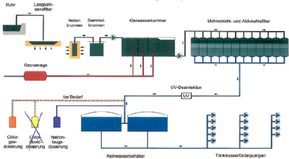
Fließschema der Aufbereitung WW Styrum-Ost
