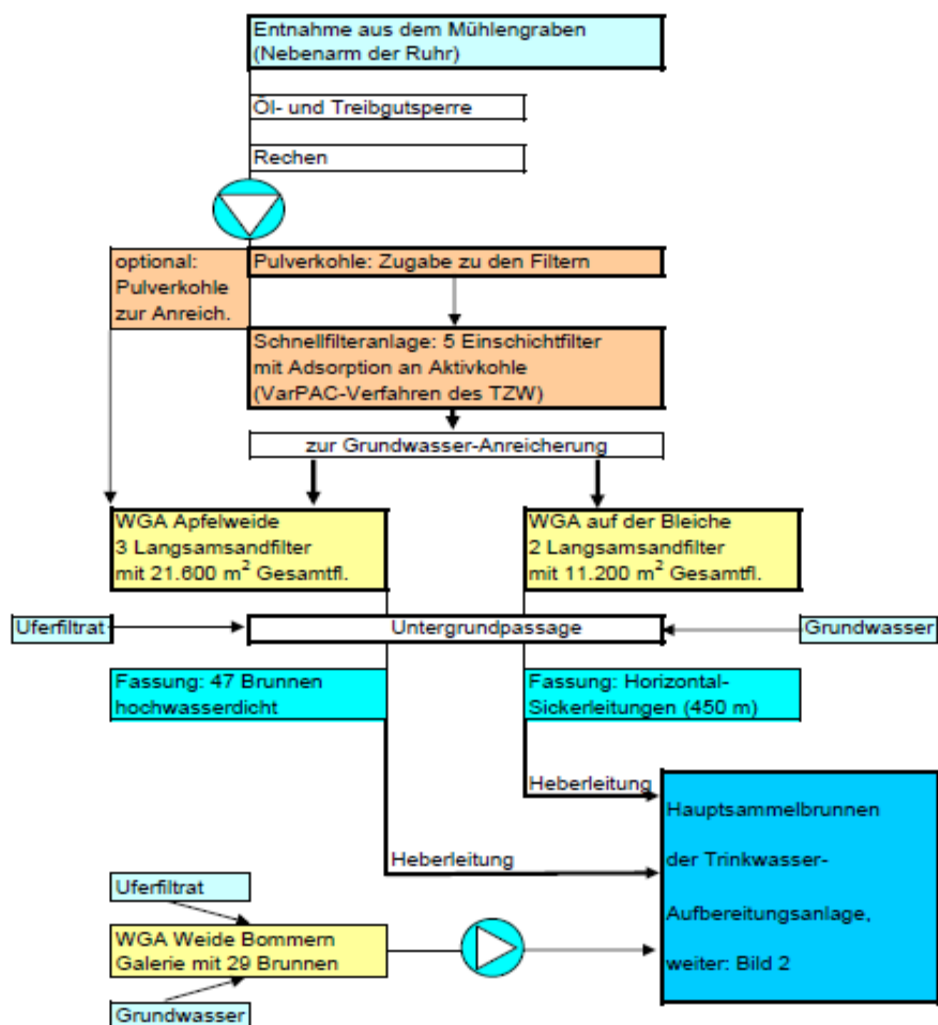
Bild 1: Gewinnung des Rohwassers einschließlich Vor-Aufbereitung des Ruhrwassers
